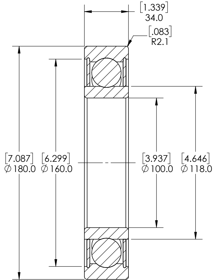
SECTION A-A
